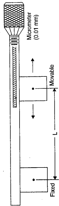
FIG. 14.55. PARALLAX BAR
